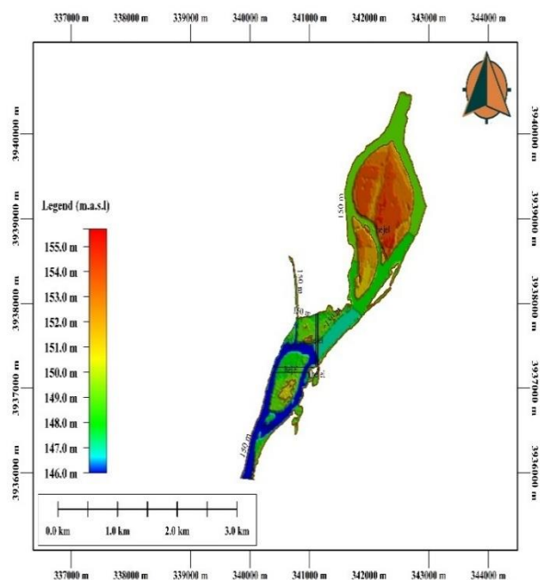
الشكل 10. شكل الخزان عند المنسوب 149م عند الموقع الثامن
