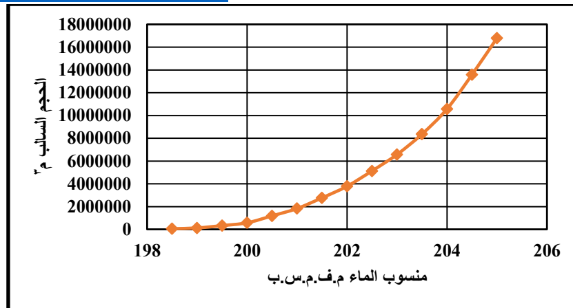
الشكل 16. العلاقة بين منسوب الماء مع الحجم السالب (حجم الخزين) في السد الثالث (حمام العليل)
