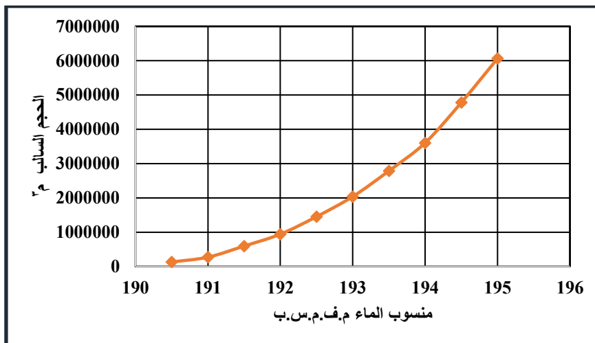
الشكل 17. العلاقة بين منسوب الماء مع الحجم السالب (حجم الخزين) في السد الرابع (منيرة)
