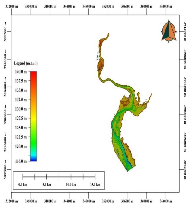
الشكل 12. شكل الخزان عند المنسوب 130م عند الموقع العاشر
