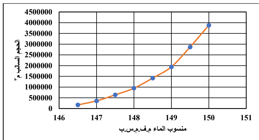
الشكل 21. العلاقة بين منسوب الماء مع الحجم السالب في السد الثامن (الهيكل)
