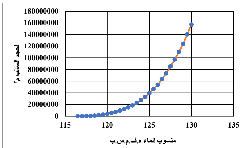
الشكل 23. العلاقة بين منسوب الماء مع الحجم السالب في السد العاشر (مكحول)
