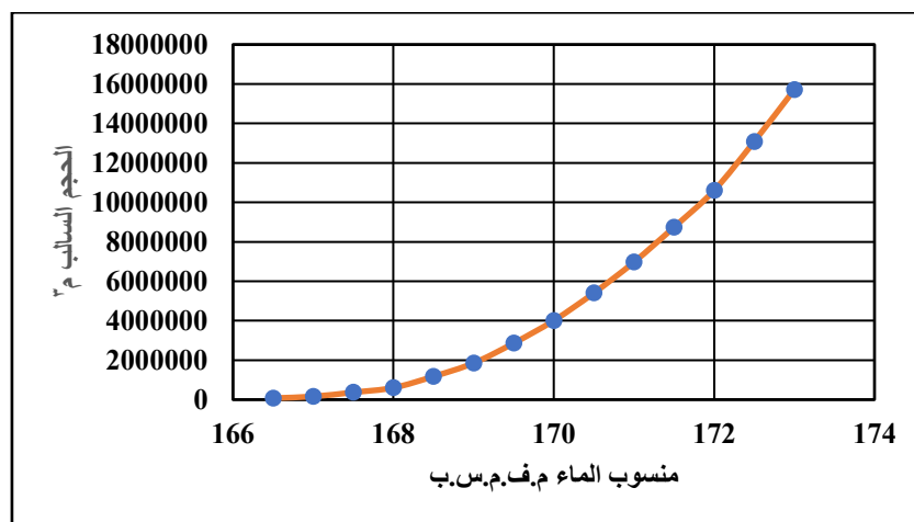
الشكل 20. العلاقة بين منسوب الماء مع الحجم السالب (حجم الخزين) في السد السابع (القيارة)
