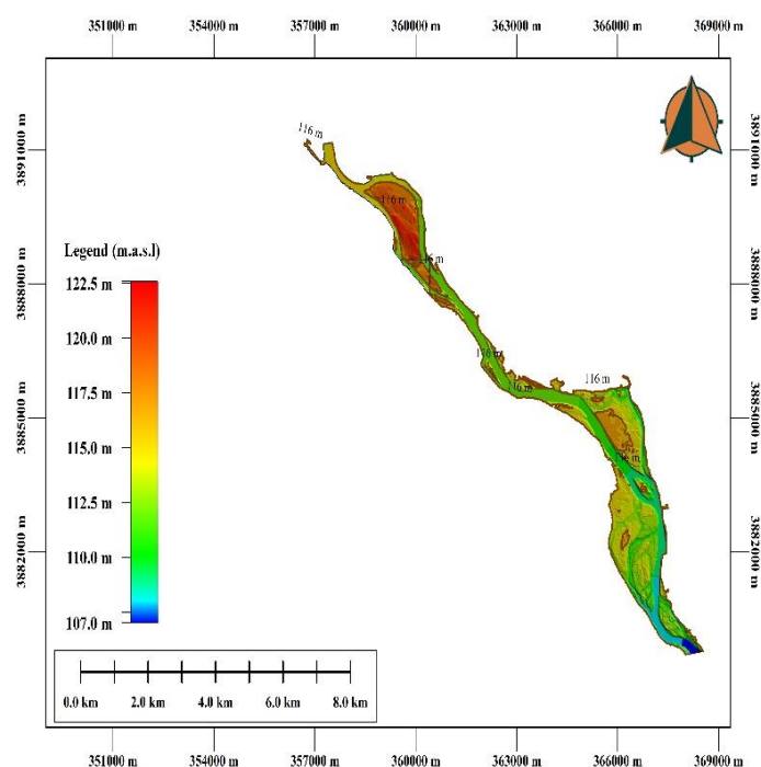
الشكل (14). شكل الخزان عند المنسوب 116م عند الموقع الحادي عشر
