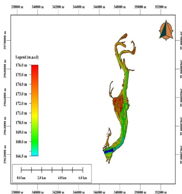
الشكل 9. شكل الخزان عند المنسوب 173م عند الموقع السابع
