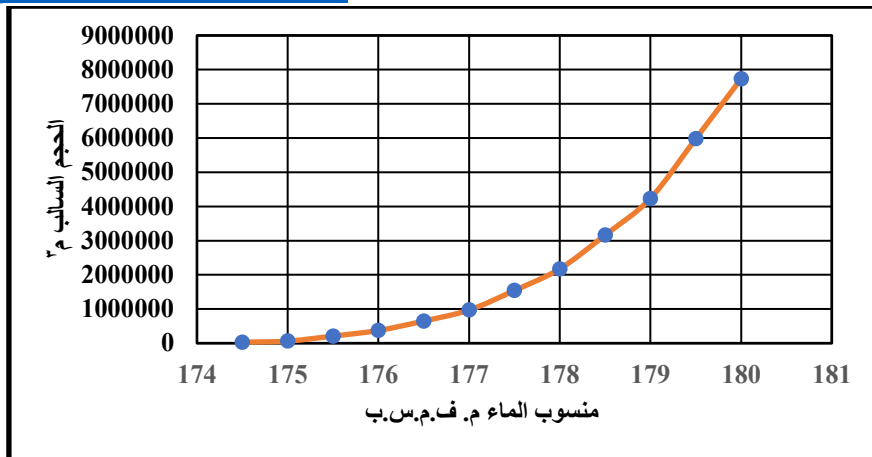
الشكل 19. العلاقة بين منسوب الماء مع الحجم السالب في السد السادس (الزوية)
