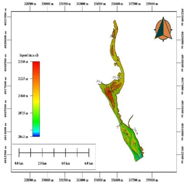
الشكل 4. شكل الخزان عند المنسوب 211,5م عند الموقع الثاني
