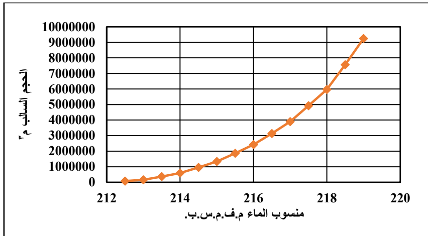
الشكل 13. العلاقة بين منسوب الماء مع الحجم السالب (حجم الخزين) لخزان السد الأول (الجسر القديم).
