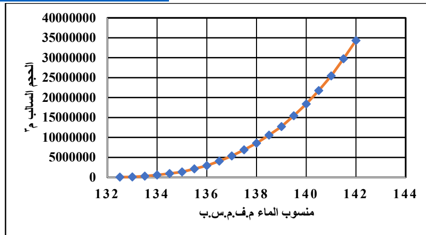
الشكل 22. العلاقة بين منسوب الماء مع الحجم السالب في السد التاسع (شاطي الجدر)
