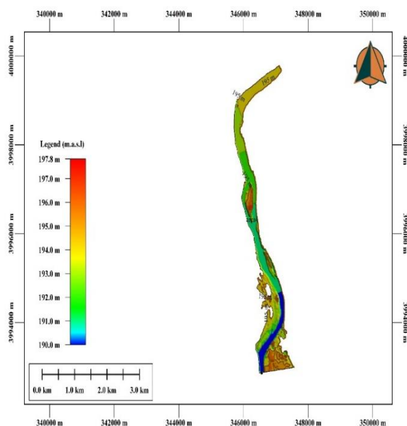
الشكل 6. شكل الخزان عند المنسوب 195م عند الموقع الرابع
