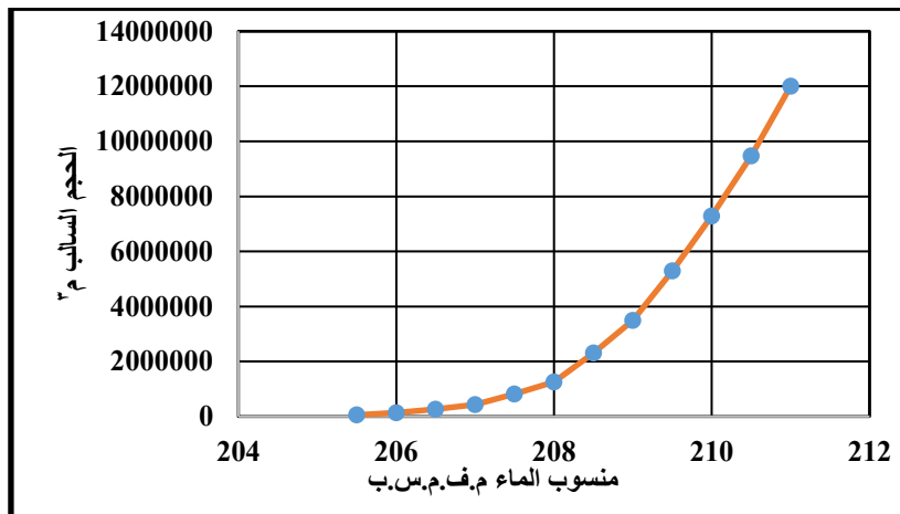
الشكل 15. العلاقة بين منسوب الماء مع الحجم السالب (حجم الخزين) في السد الثاني (الجماسة)
