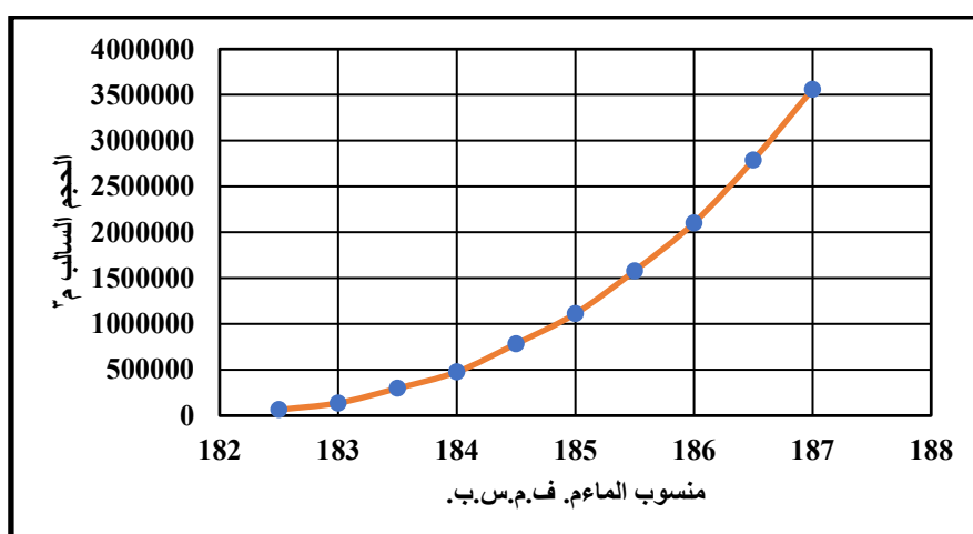
الشكل 18. العلاقة بين منسوب الماء مع الحجم السالب (حجم الخزين) في السد الخامس (السفينة)
