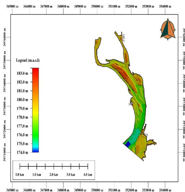
الشكل 8. شكل الخزان عند المنسوب 180م عند الموقع السادس
