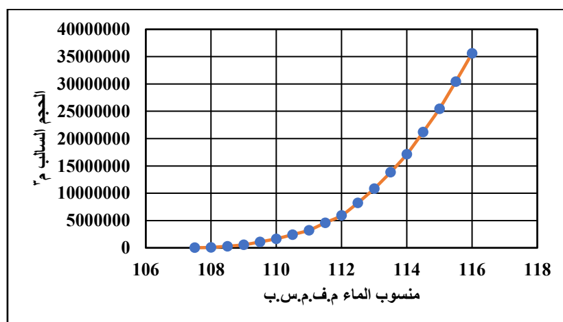
الشكل 24. العلاقة بين منسوب الماء مع الحجم السالب في السد الحادي عشر (الفتحة)
